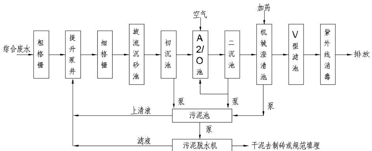
图 5.2.1-1 金西污水处理一期工程工艺流程
