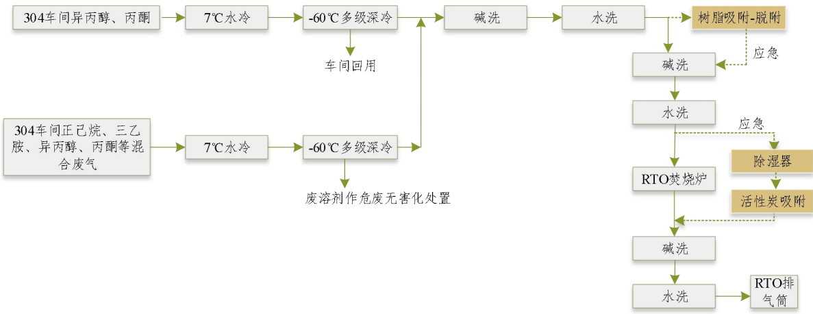
图 7.2-2 本项目车间工艺废气预处理流程
