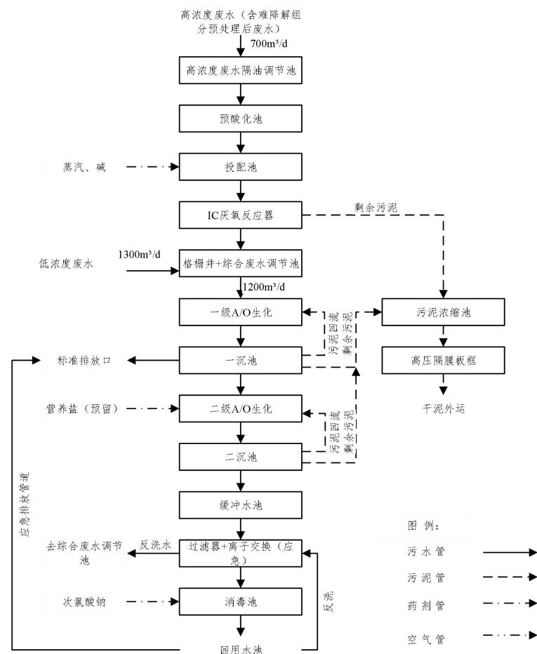
图 7.1-2 本项目废水处理工艺流程图
