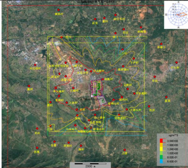
图 6.1.6-4 正己烷叠加后日平均质量浓度分布图
